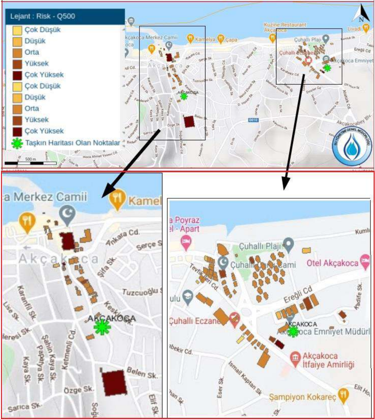
Şekil 2. 15. Akçakoca İlçesi Q500 Taşkın Risk Haritası ( http://taskinyonetimportal.tarimorman.gov.tr )
